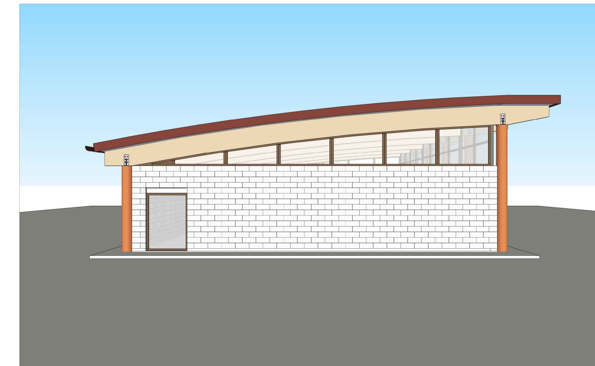
RENDERING PROSPETTO OVEST
